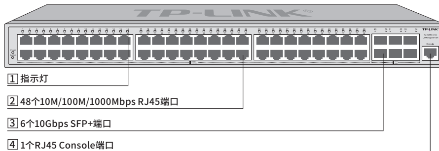
图1-1 TL-NS650-48G6T前面板示意图
